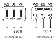
Клемная колодка
